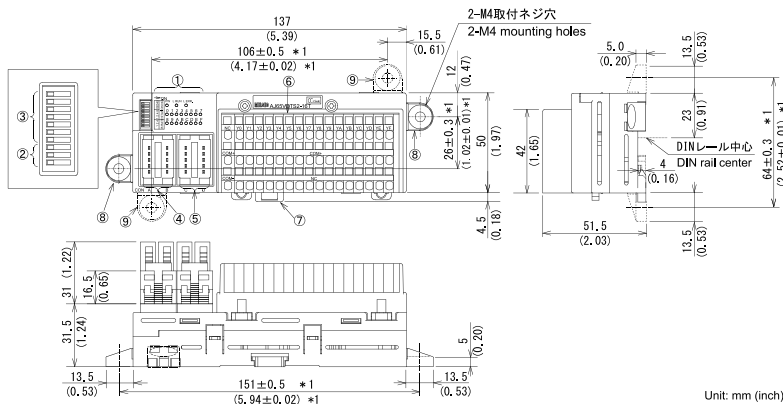
* 1 取付けネジ加工寸法 (取付ピッチ) Mounting pitch
