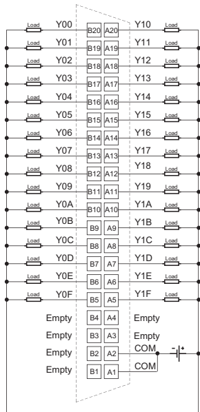
QY41H (Rated load voltage: 5 to 24VDC) (Tension nominale d'entrée 5 à 24 V ca)
