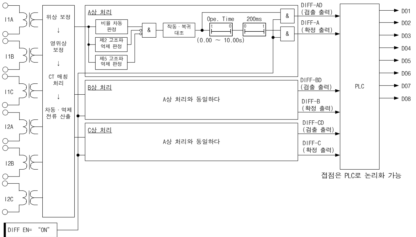
그림 3-1 전류비율 차동 요소(DIFF) 내부 기능 블록도
