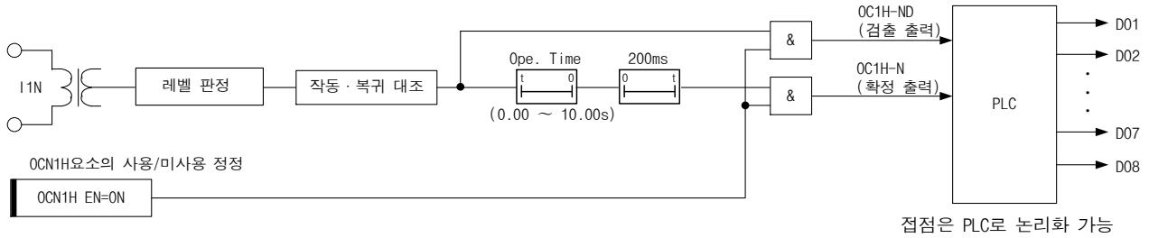
그림 3-21 OCN1H요소 내부 기능 블록도
