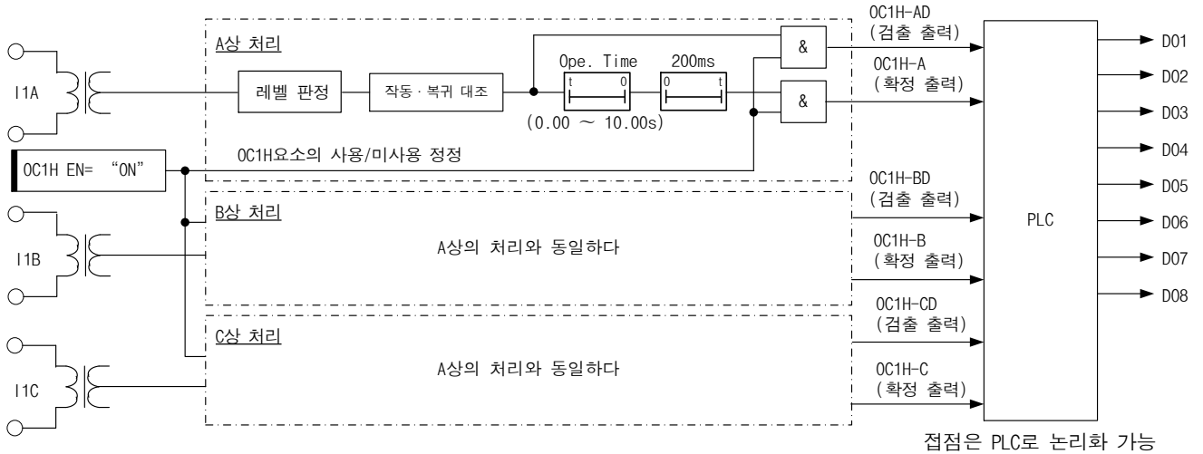
그림 3-11 과전류 순시 요소(OC1H) 내부 기능 블록도
