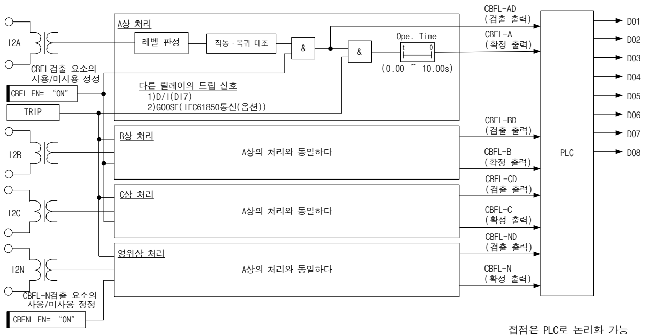
그림 3-28 CBFL 요소 내부 기능 블록도
