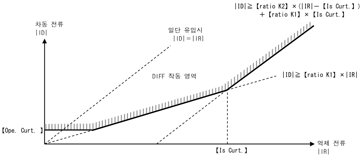
그림 3-2 전류 비을 차동 요소(DIFF)의 동작 특성
