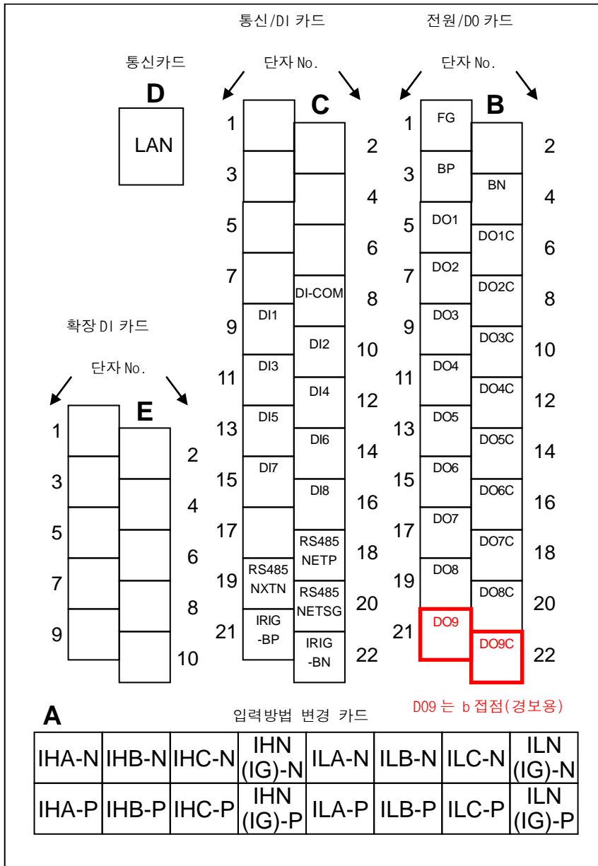
그림 7-2경보DO의 위치
