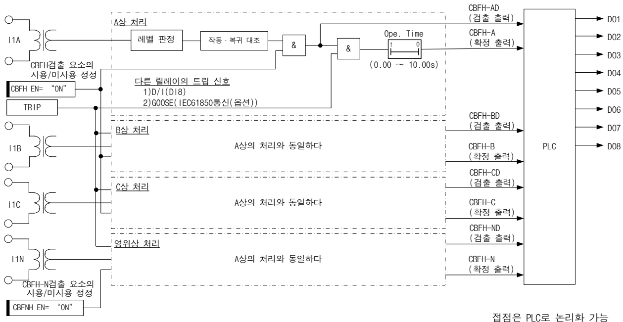
그림 3-27 CBFH 요소 내부 기능 블록도
