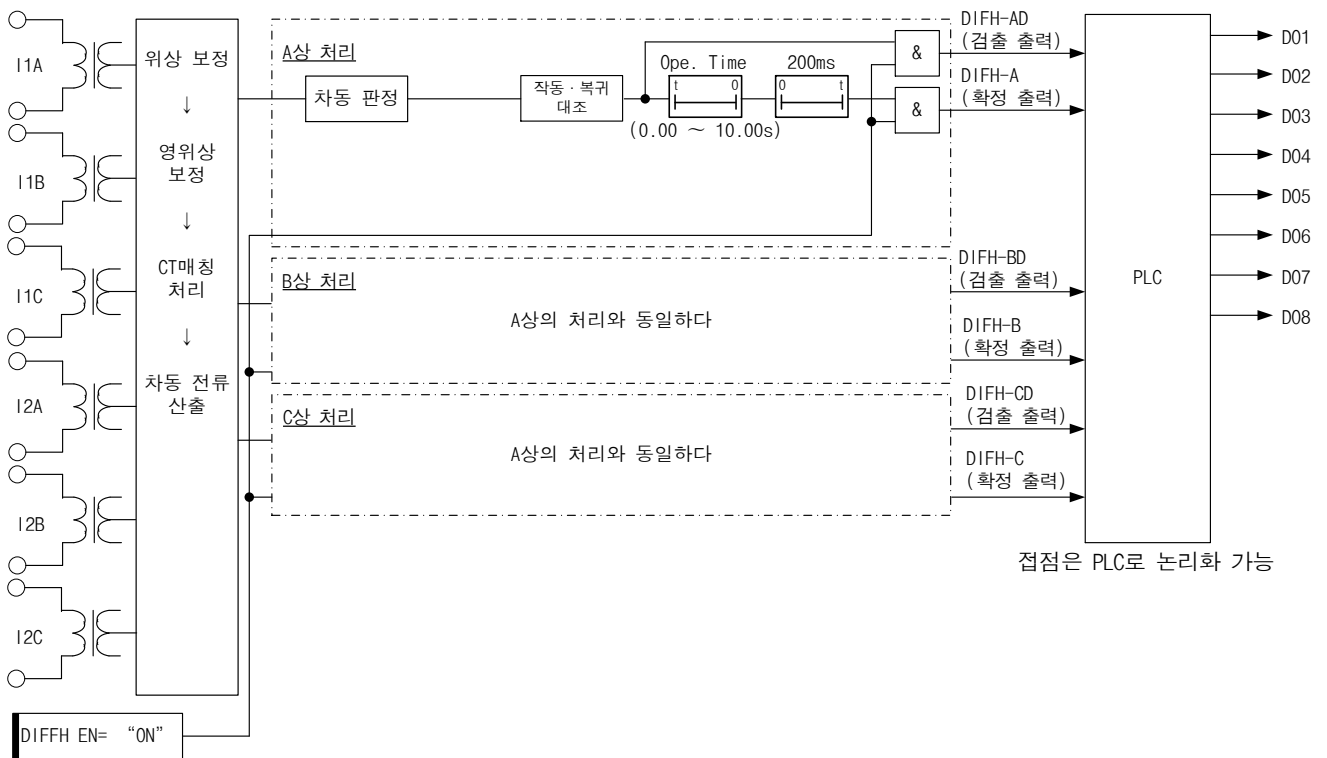
그림 3-7 차동 과전류 요소(DIFFH) 내부 기능 블록도
