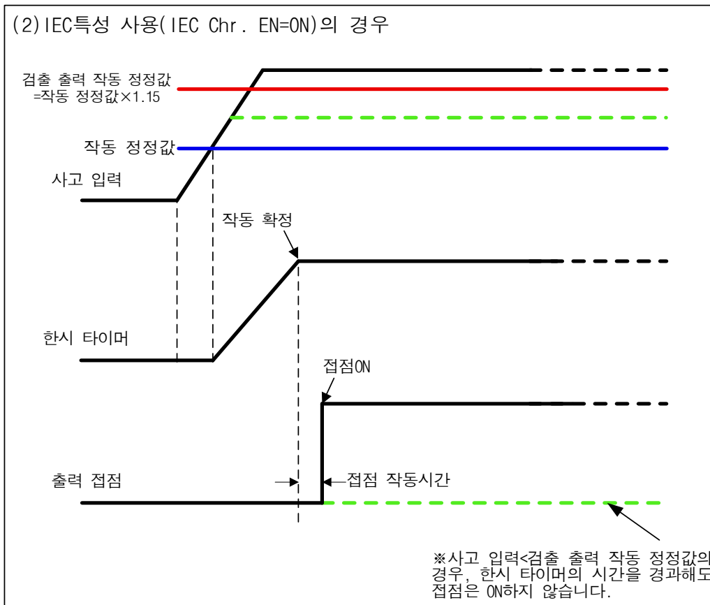
그림 3-15 OC4L요소 정정 항목
