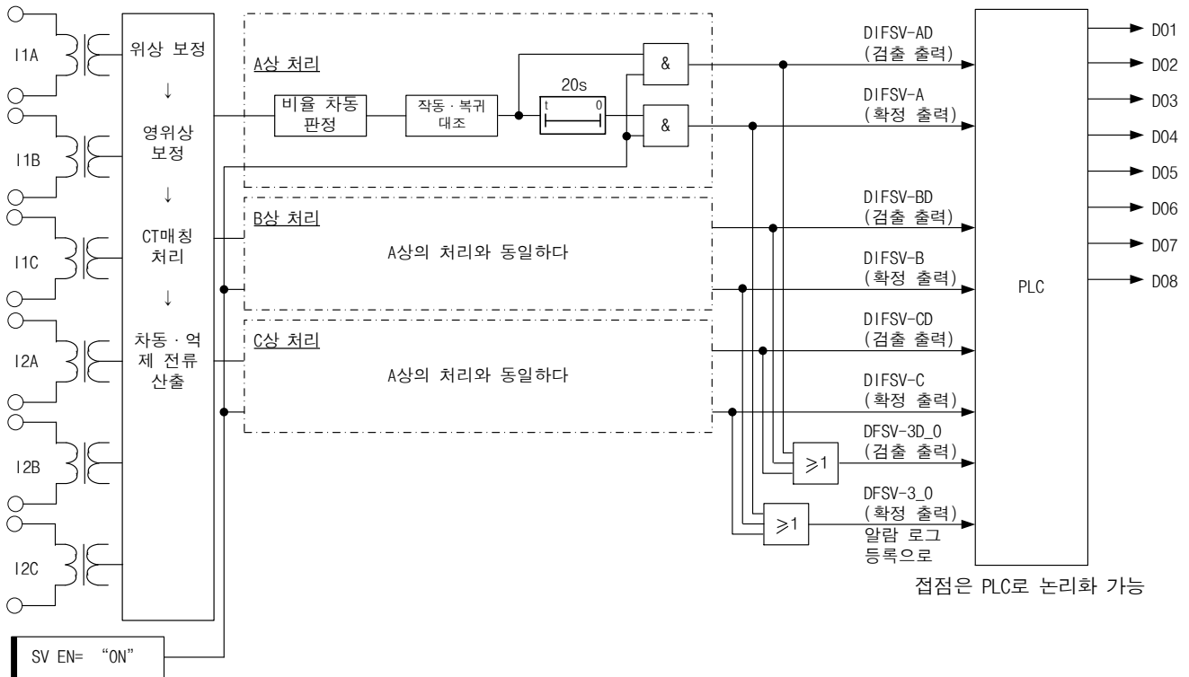
그림 3-5 전류 비율 차동 감시 요소(DIFSV) 내부 기능 블록도
