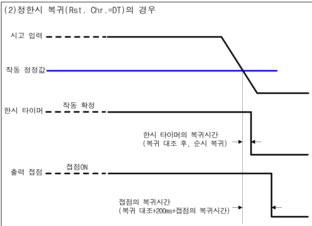
그림 3-16 복귀 시간 특성(1)
