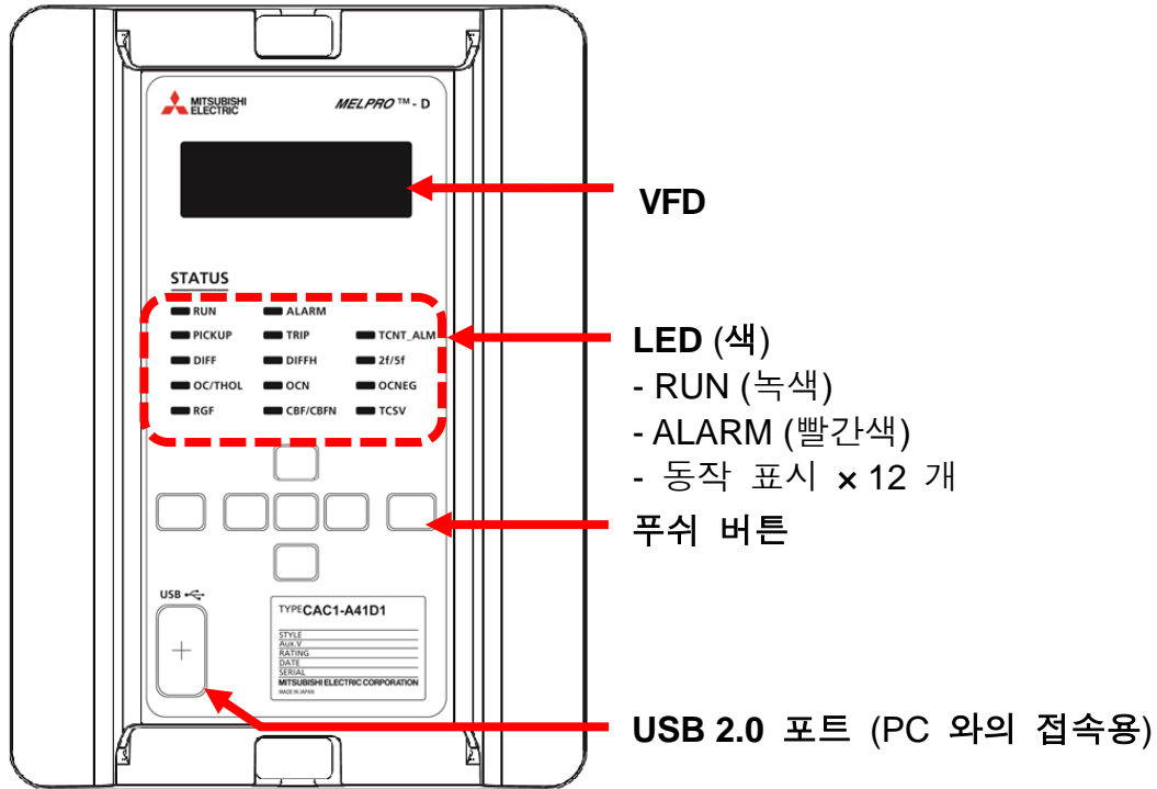
그림 1-3 릴레이 정면도
