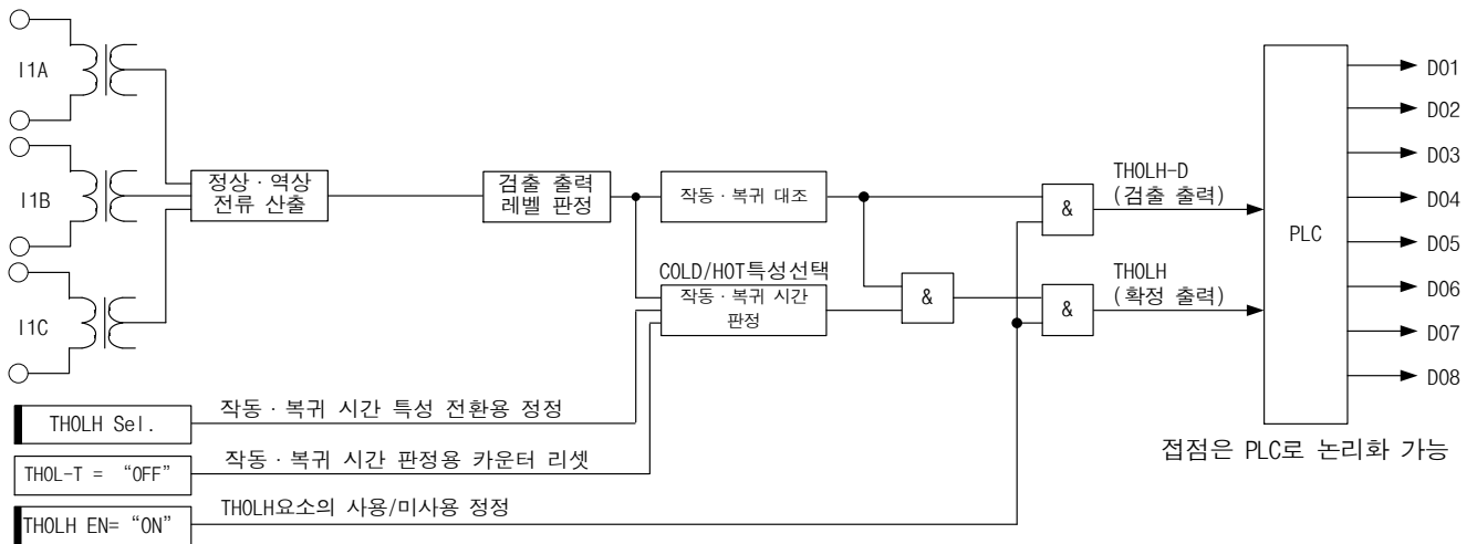
그림 3-24 THOLH 요소 내부 기능 블록도
