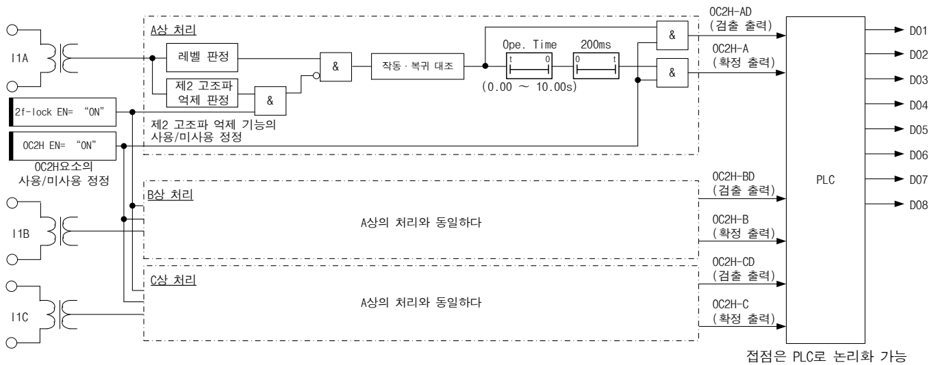
그림 3-12 OC2H요소 내부 기능 블록도
