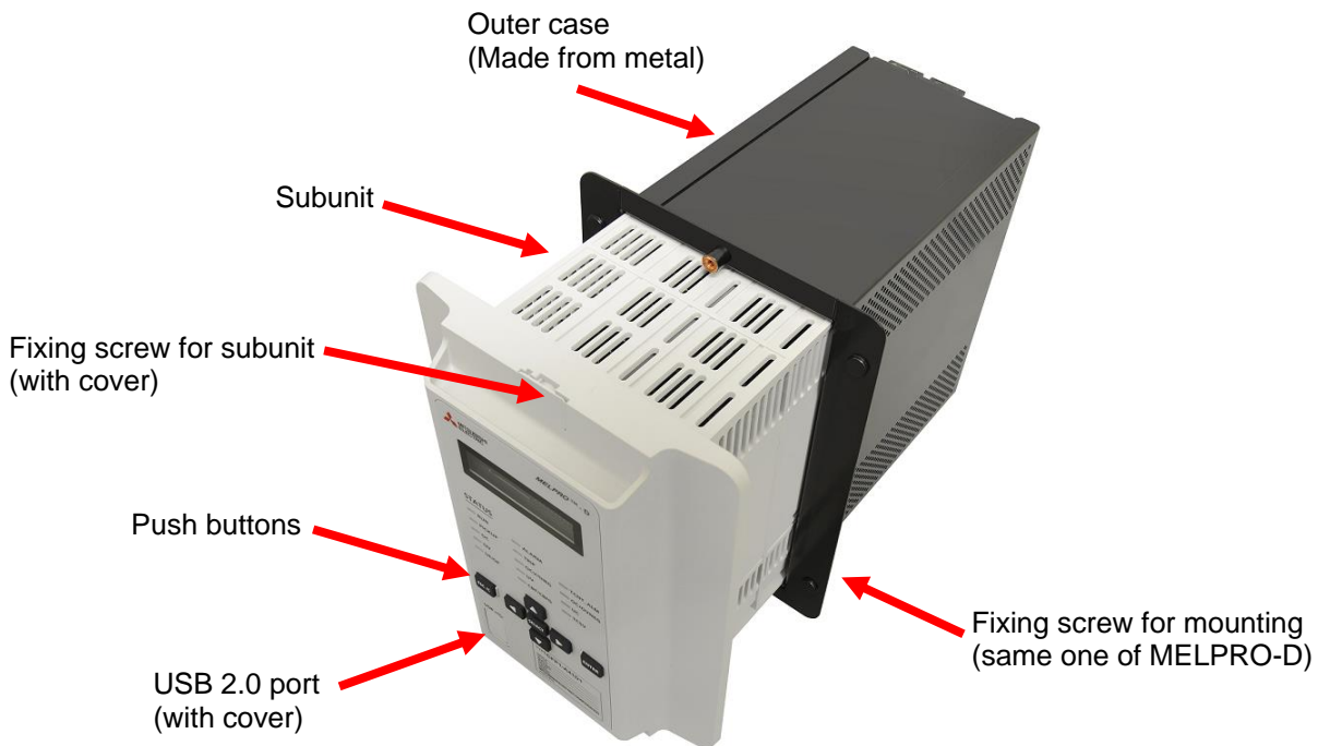
그림 1-5 릴레이 외관도
