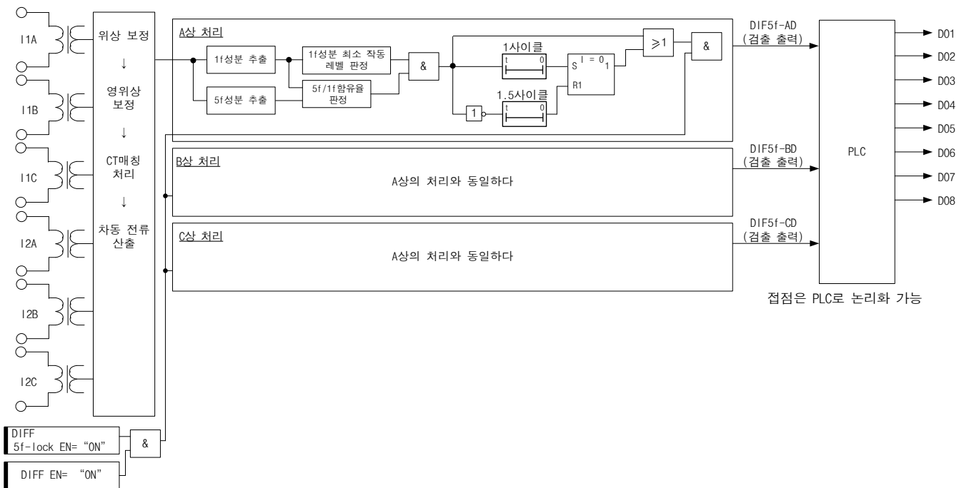
그림 3-4 제5 고조파 억제 기능(차동 전류) 내부 블록도
