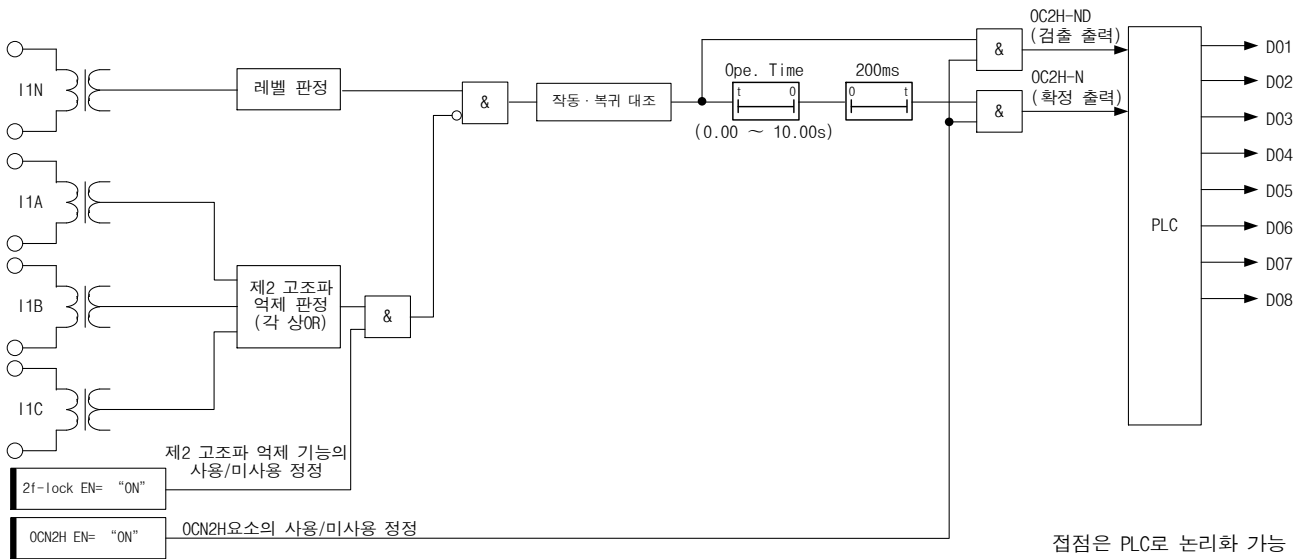
그림 3-22 OCN2H요소 내부 기능 블록도
