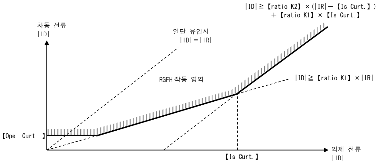
그림 3-9 영상 전류 비율 차동 요소(RGFH)의 동작 특성
