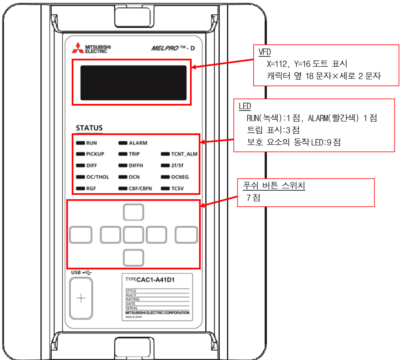
그림 4-1 정면 패널 각부 설명
