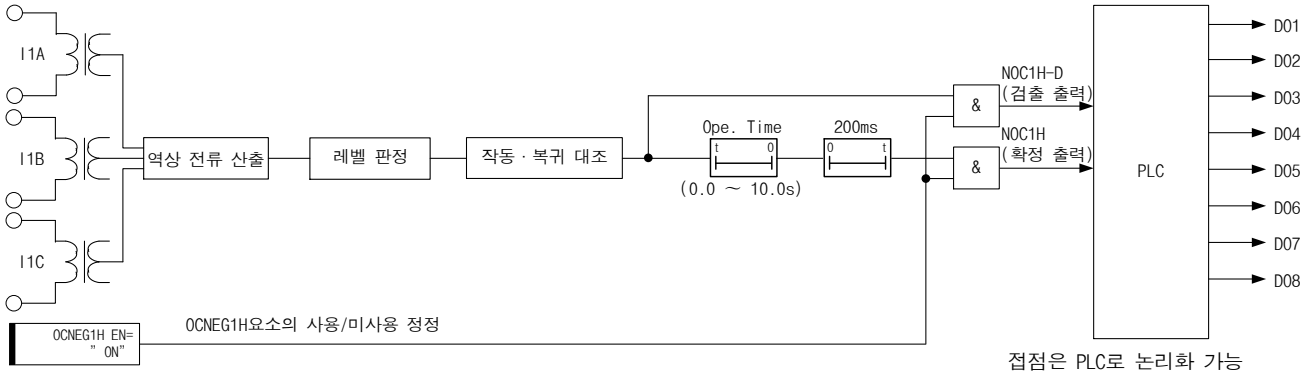
그림 3-26 OCNEG1H요소 내부 기능 블록도
