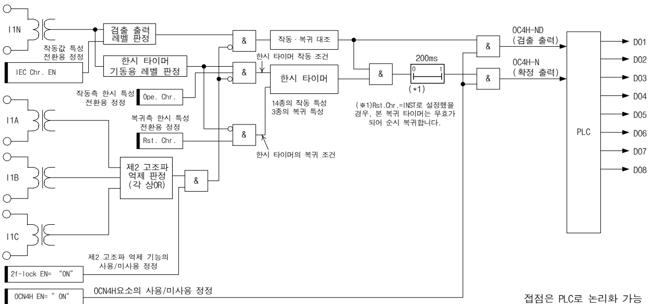
그림 3-23 OCN4H요소 내부 기능 블록도
