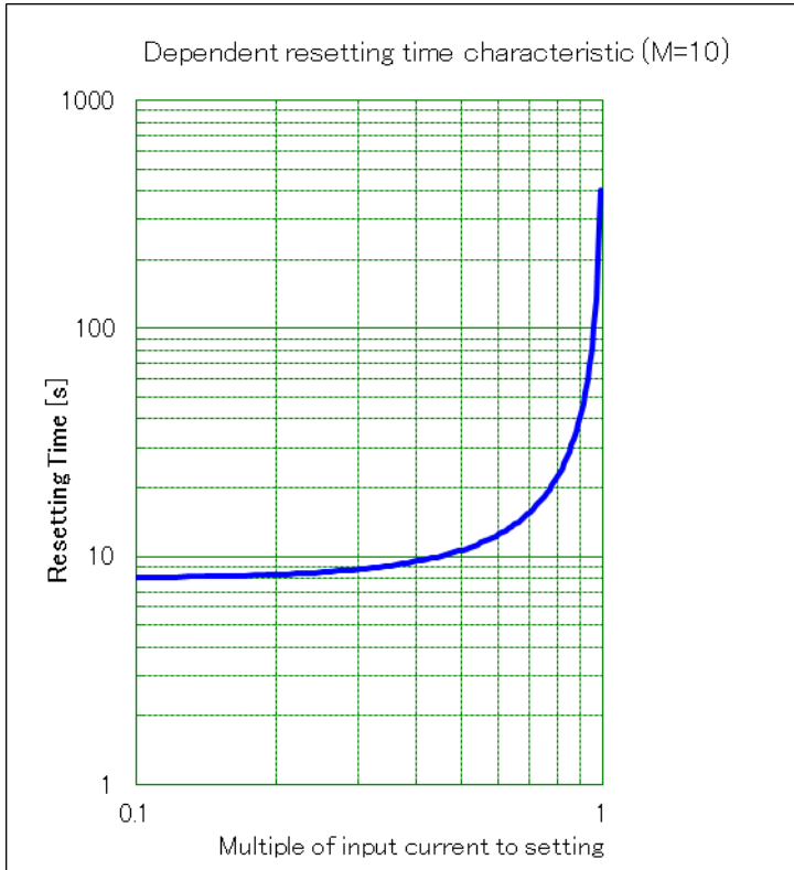
그림 3-20 복귀 시간 특성
