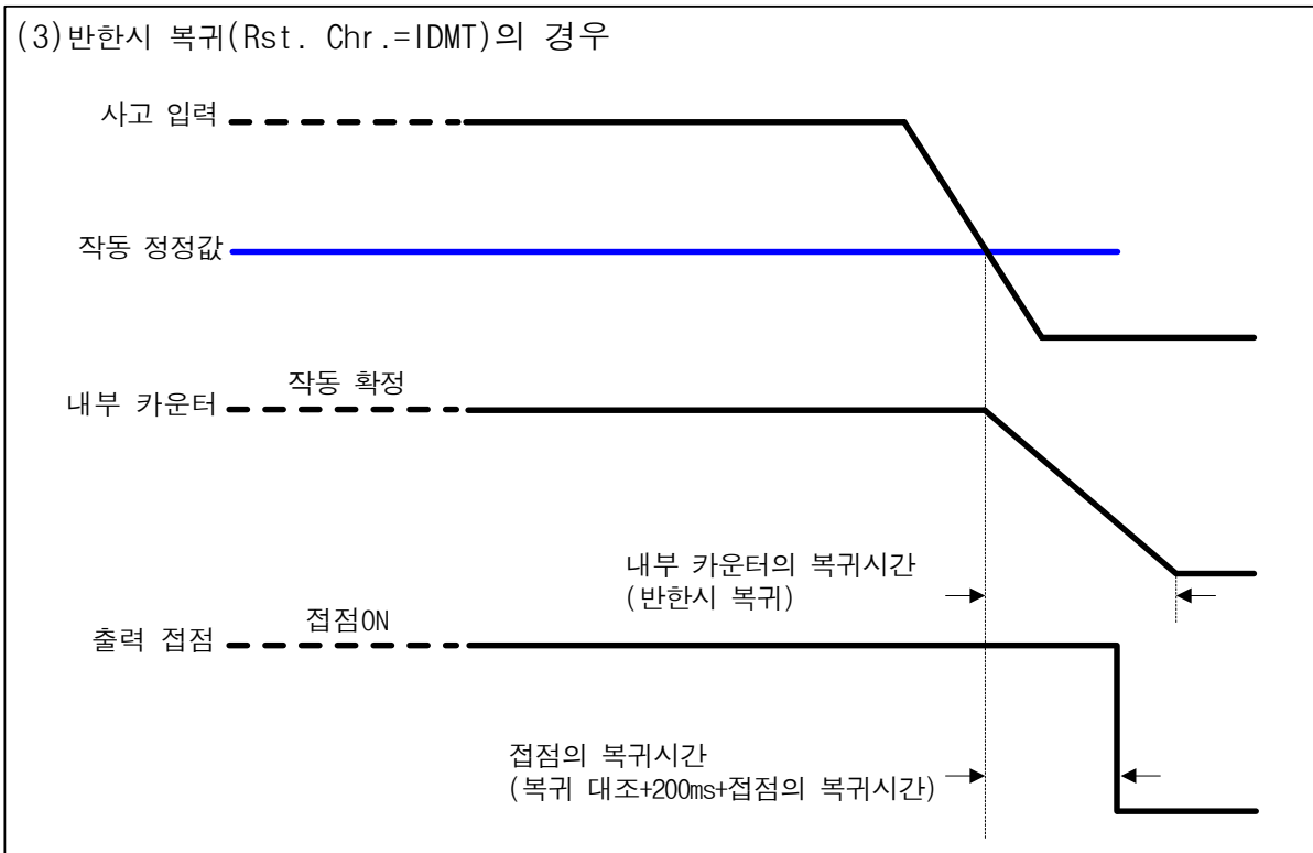
그림 3-17 복구 시간 특성(2)
