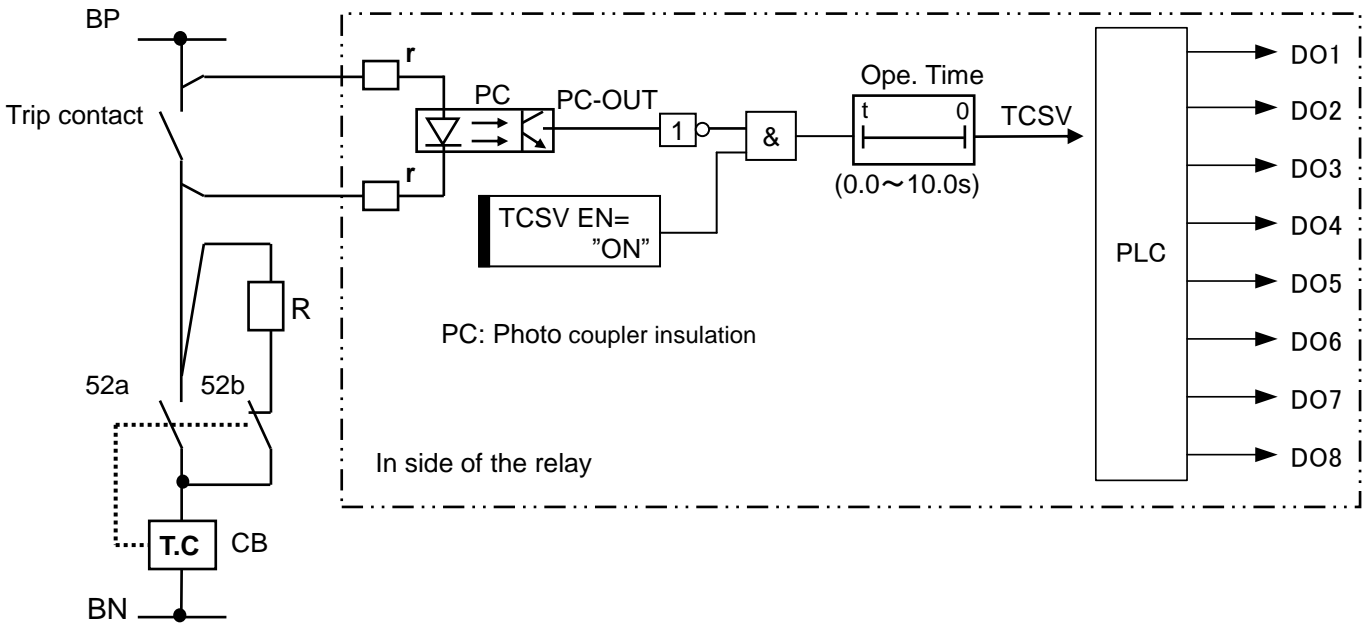
그림 3-29 트립코일 감시 회로
