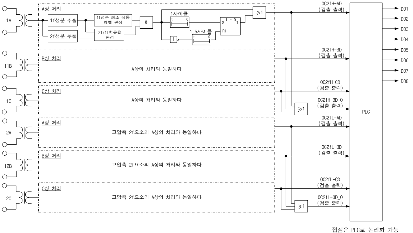
그림 3-13 제2 고조파 억제 기능 내부 블록도
