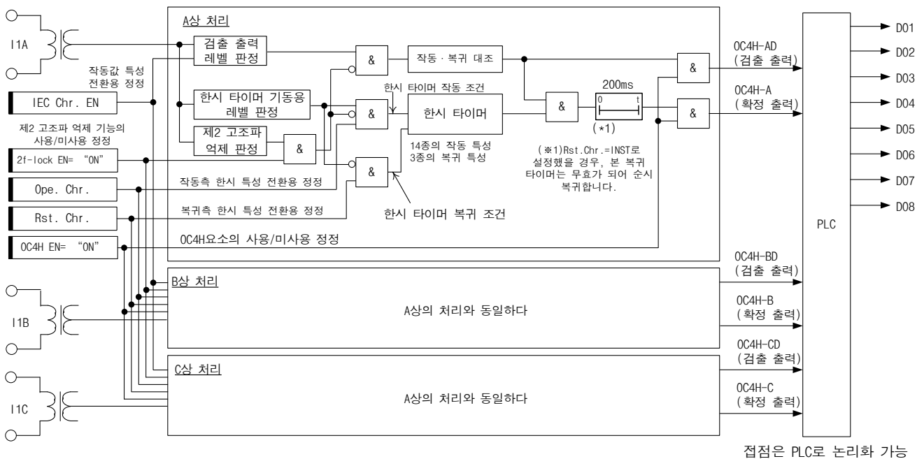
그림 3-14 OC4H요소 내부 기능 블록도
