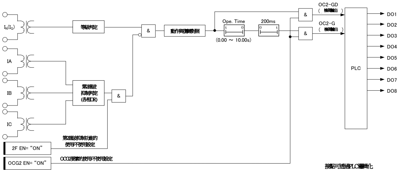
圖 3-13 OCG2要素 內部功能區塊圖
