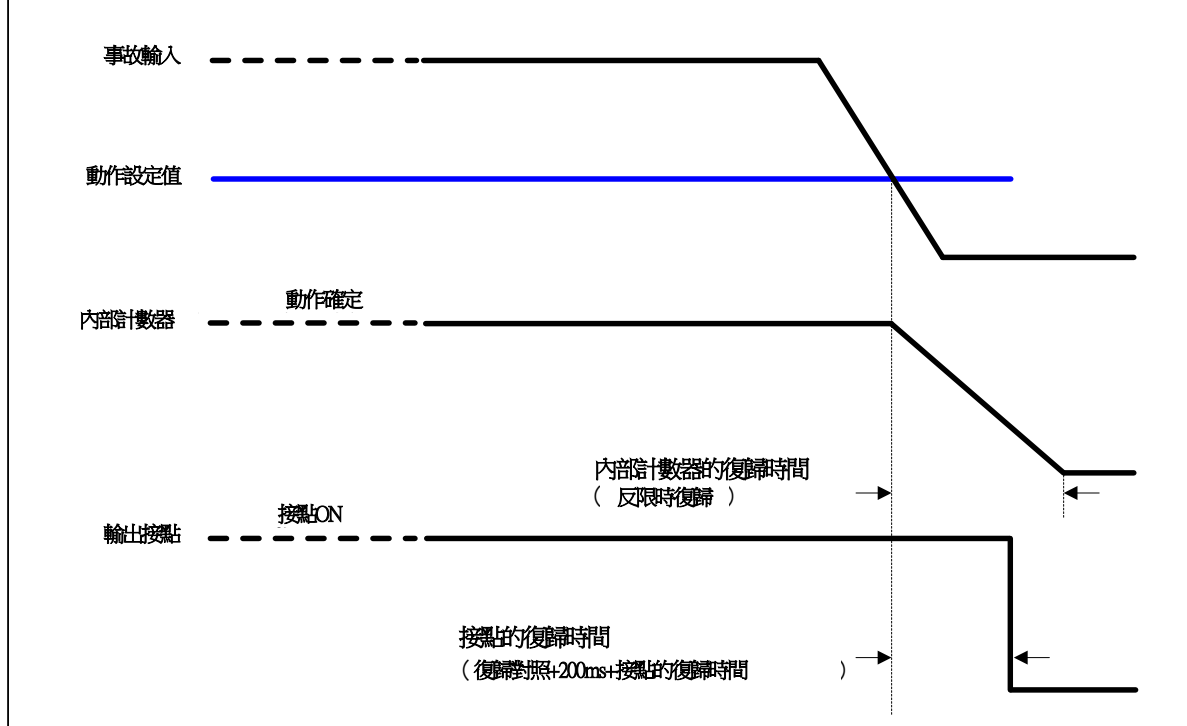
圖 3-8 復歸時間特性(2)
