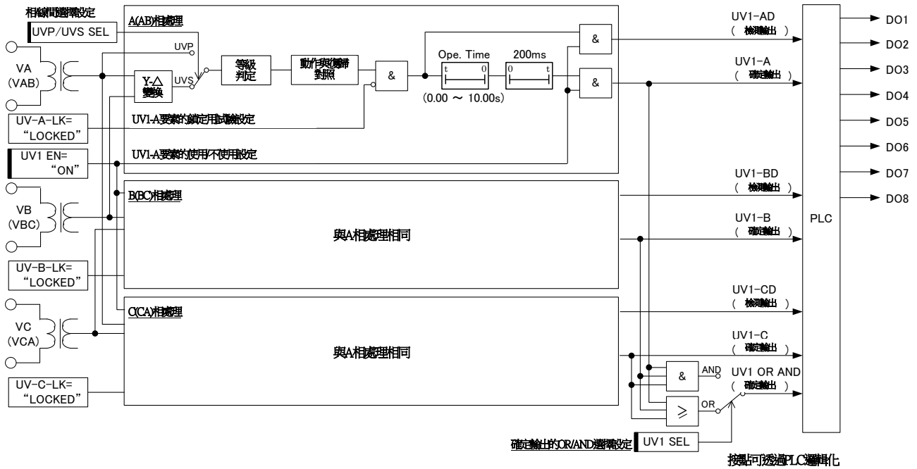
圖 3-22 UV1要素 內部功能區塊圖
