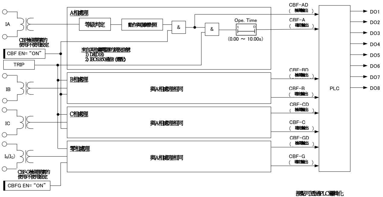
圖 3-18 CBF要素 內部功能區塊圖
