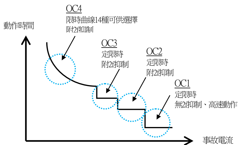
圖 3-1 過電流要素的動作時限協調曲線範例
