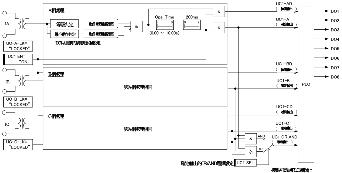
圖 3-17 UC1要素(方式2) 內部功能區塊圖
