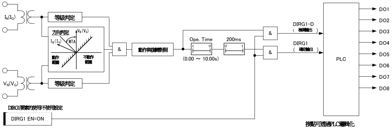
圖 3-19 DIRG1要素 內部功能區塊圖
