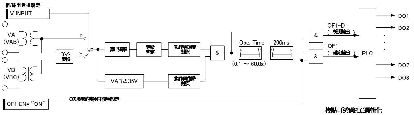
圖 3-27 OF1要素 內部功能區塊圖
