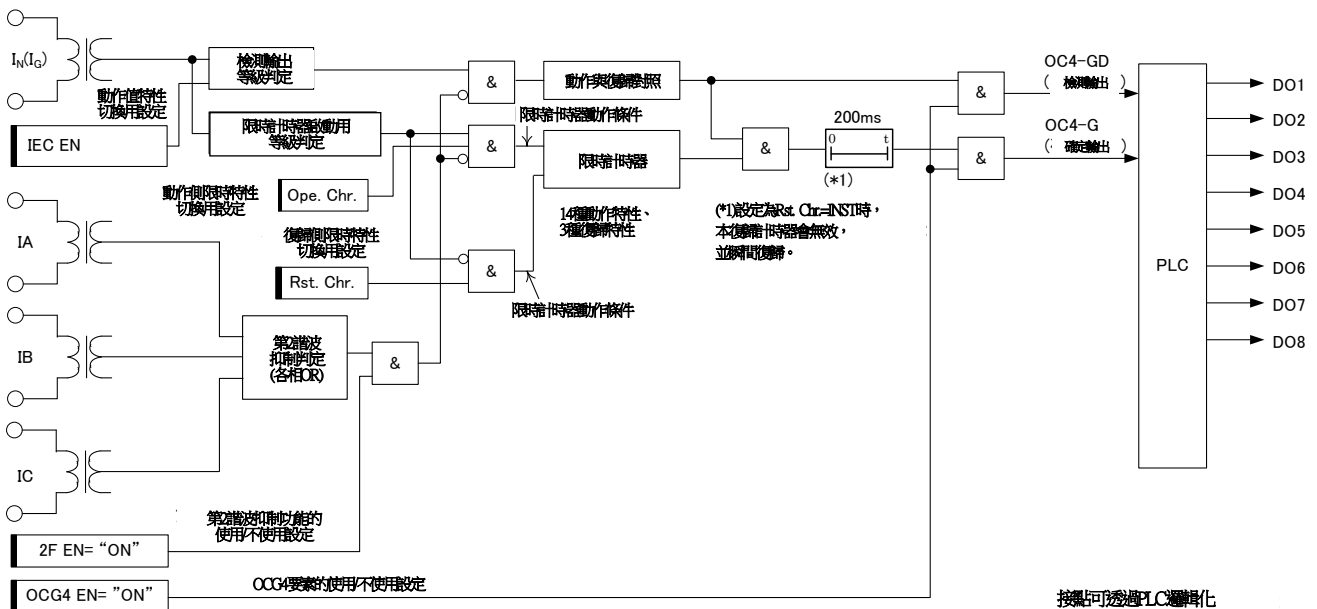
圖 3-14 OCG4要素 內部功能區塊圖
