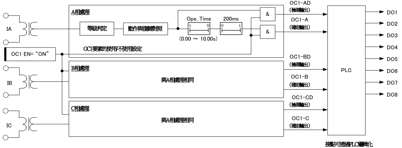
圖 3-2 過電流瞬時要素 (OC1) 內部功能區塊圖
