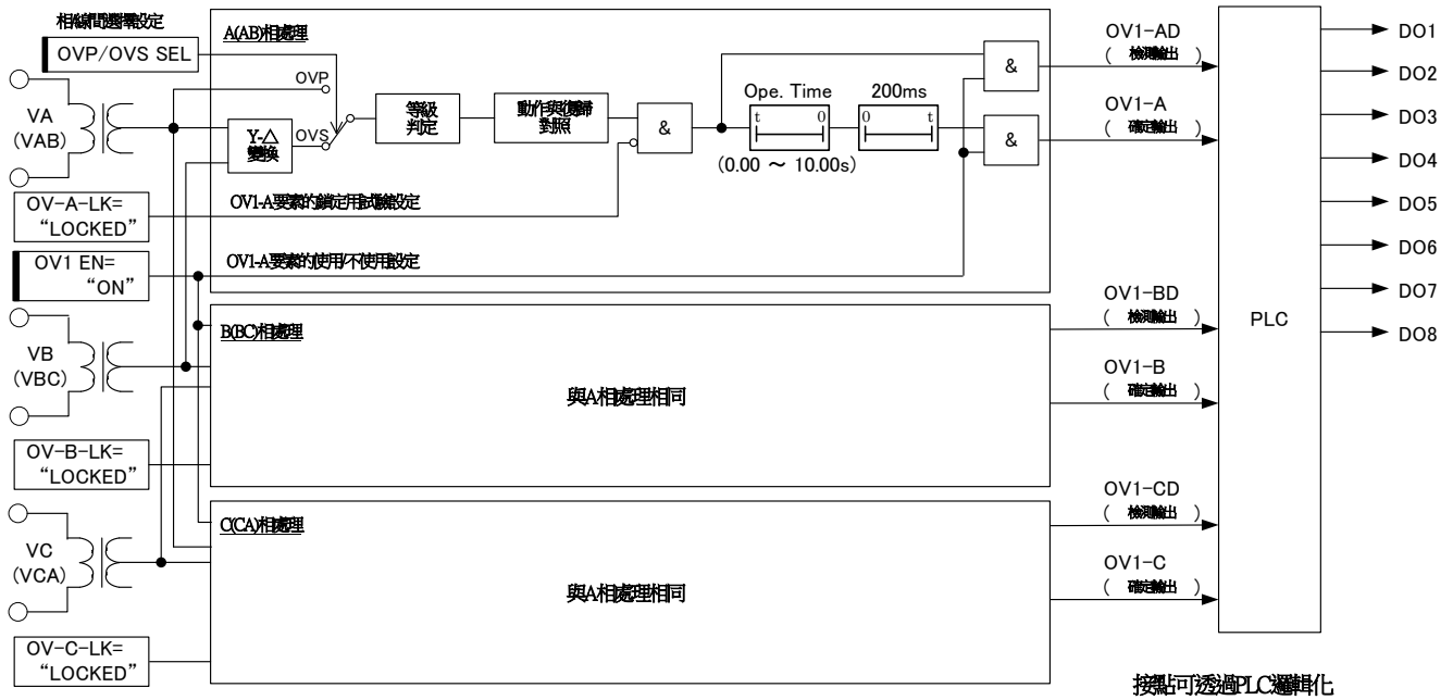
圖 3-23 OV1要素 內部功能區塊圖
