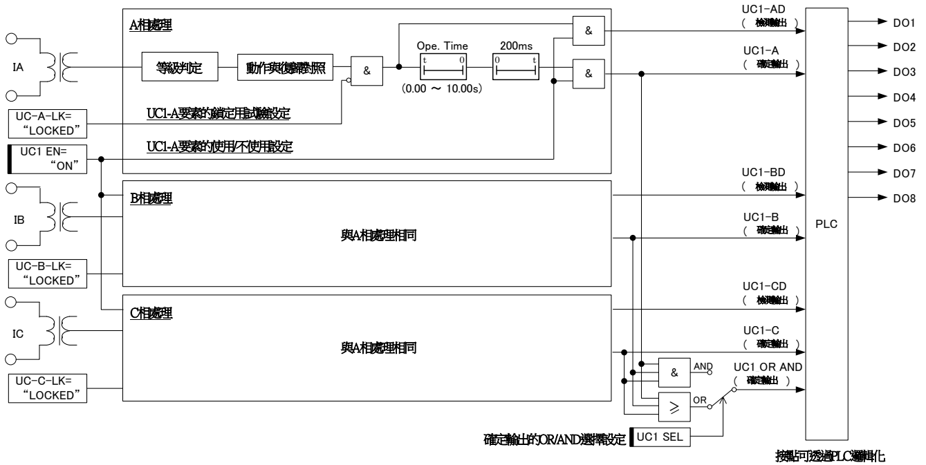
圖 3-16 UC1要素(方式1) 內部功能區塊圖
