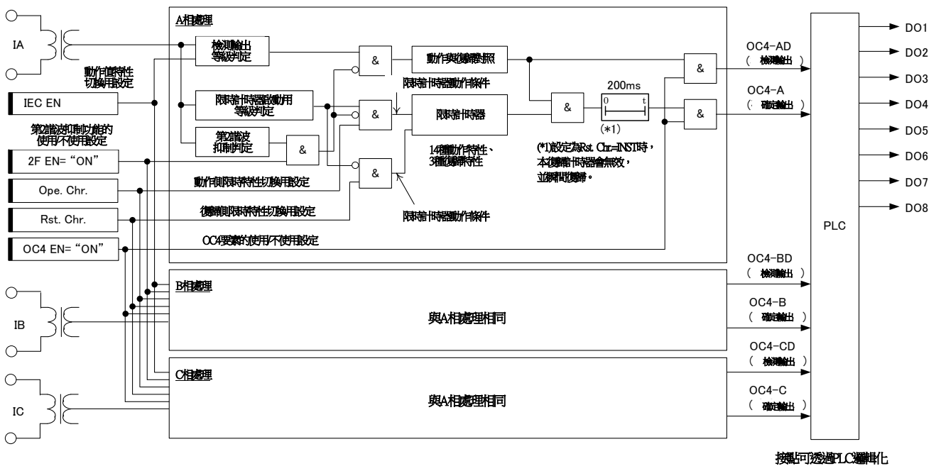
圖 3-5 OC4要素 內部功能區塊圖
