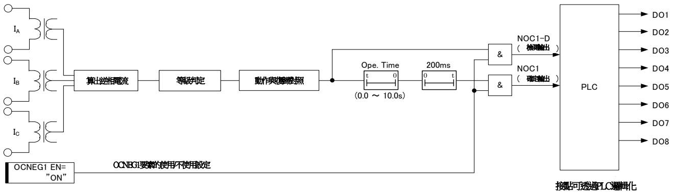
圖 3-15 OCNEG1要素 內部功能區塊圖
