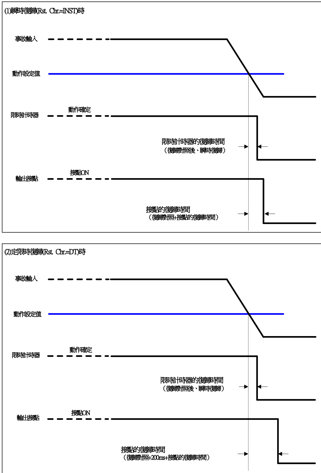
圖 3-7 復歸時間特性(1)
