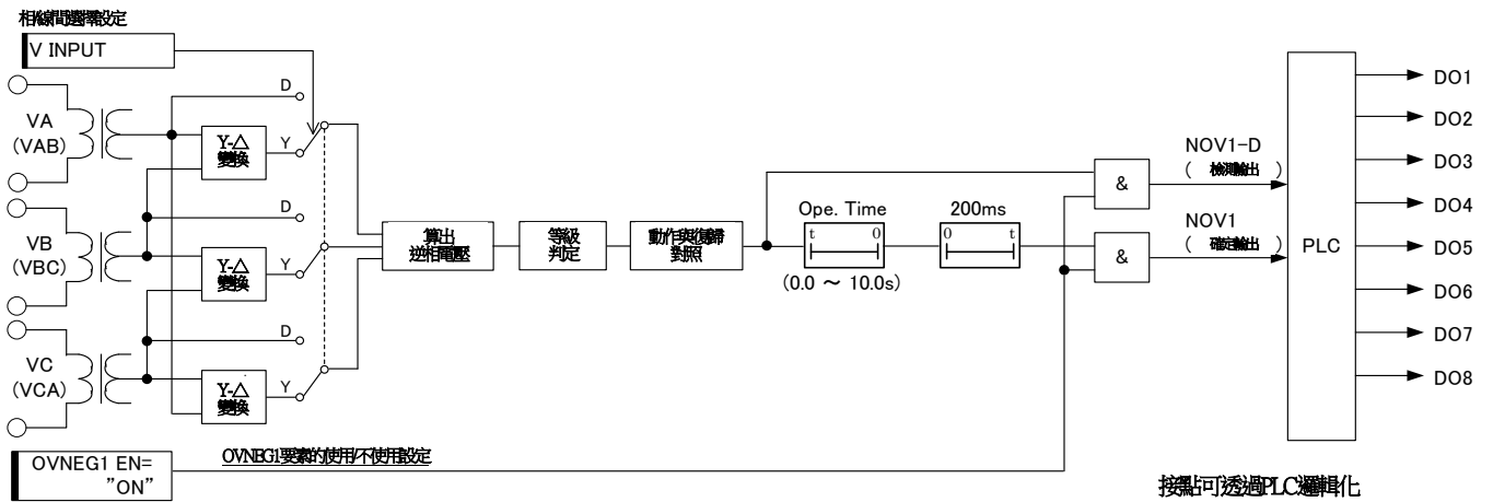
圖 3-25 OVNEG1要素 內部功能區塊圖
