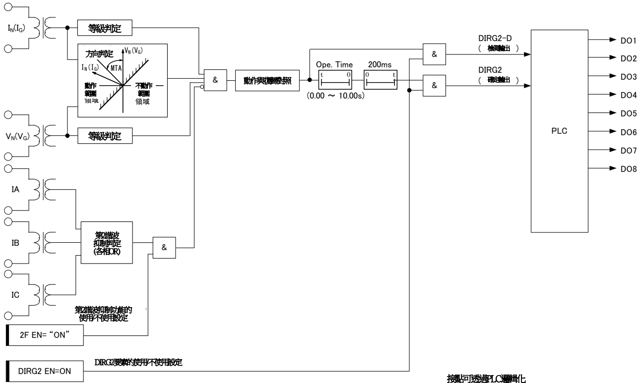
圖 3-20 DIRG2要素 內部功能區塊圖
