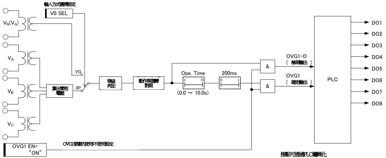
圖 3-24 OVG1要素 內部功能區塊圖
