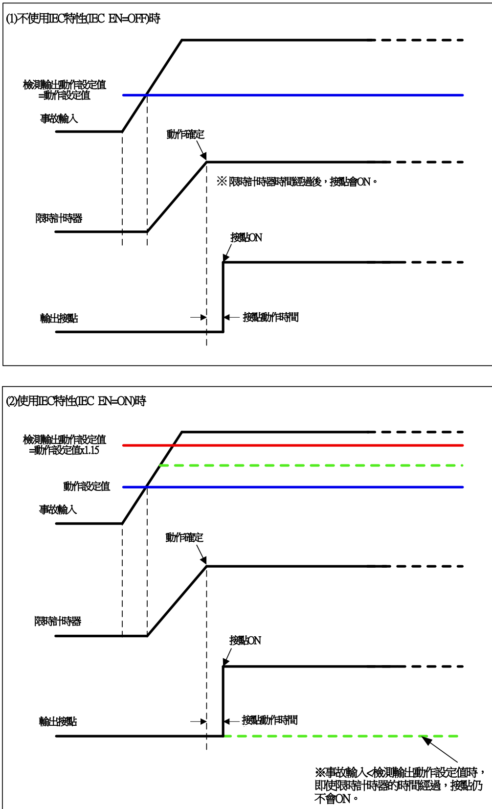
圖 3-6 有無IEC特性的比較
