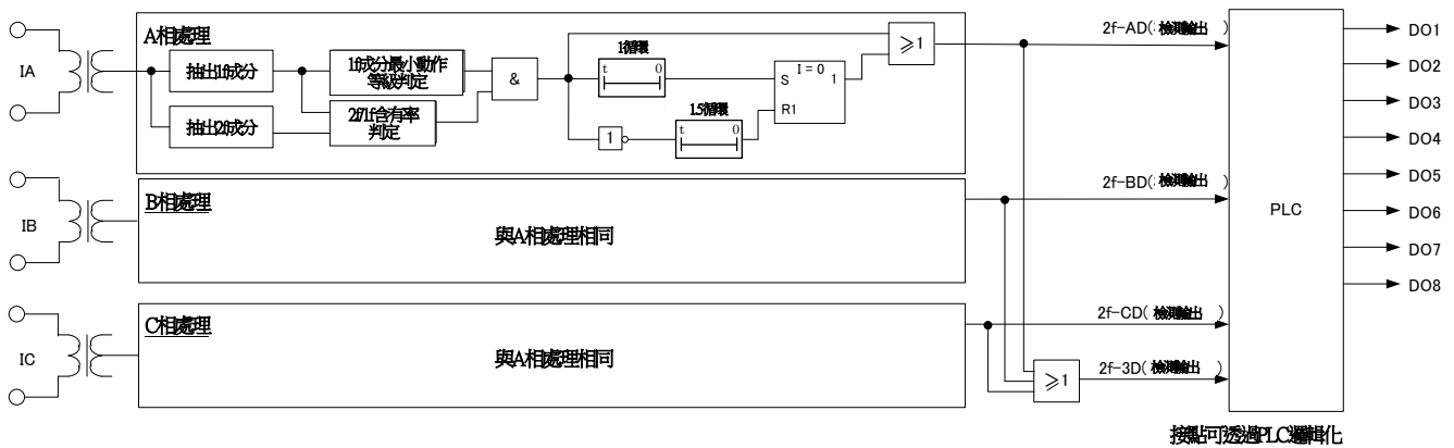
圖 3-4 第2諧波抑制功能 內部區塊圖
