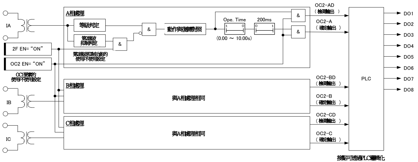
圖 3-3 OC2要素 內部功能區塊圖
