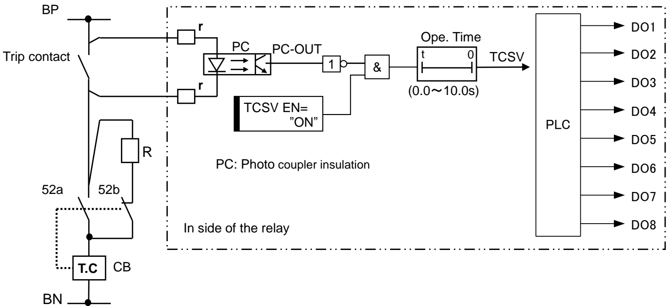
圖 3-28 跳脫線圈監控迴路
