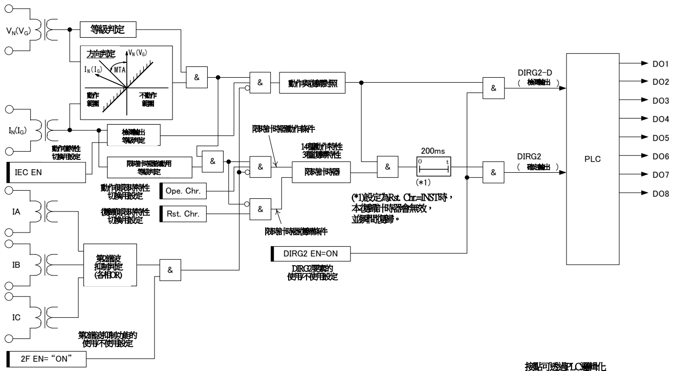
圖 3-21 DIRG4要素 內部功能區塊圖
