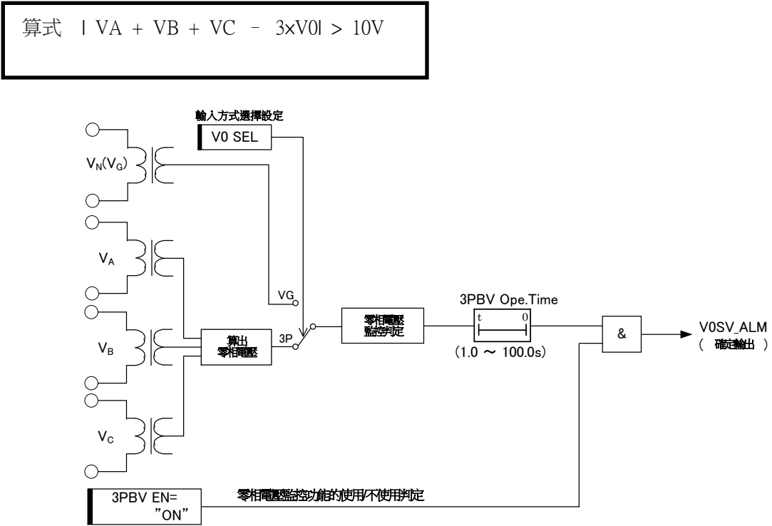
圖 3-29 零相電壓監控要素 內部功能區塊圖
