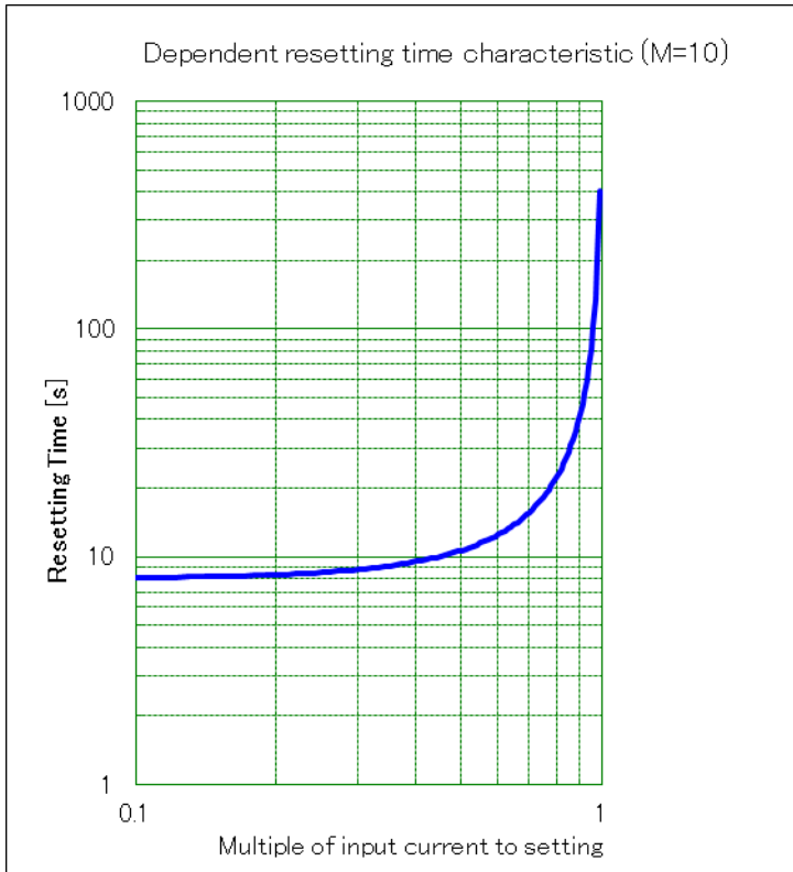
圖 3-11 復歸時間特性
