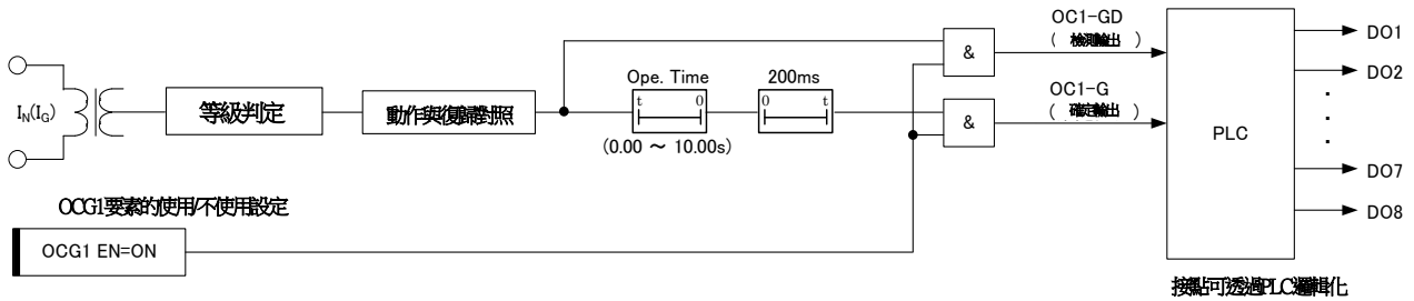
圖 3-12 OCG1要素 內部功能區塊圖
