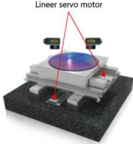
Hızalama sistemi
