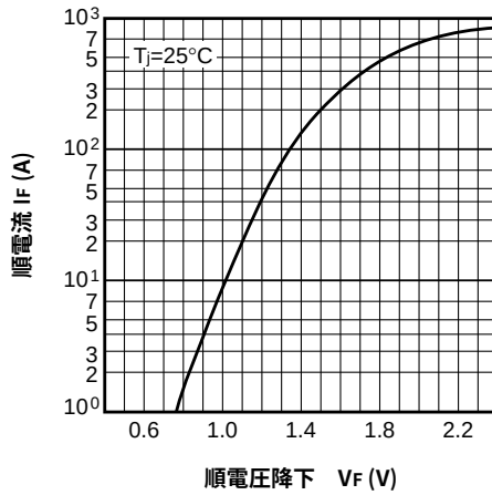
最大順特性
