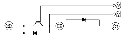
接続図 CIRCUIT DIAGRAM
