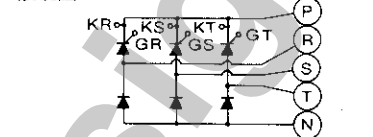
接続図
