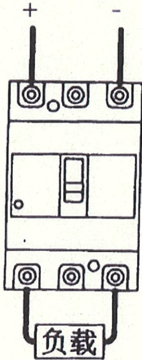
3P外形
