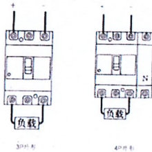
直流接线方式:
